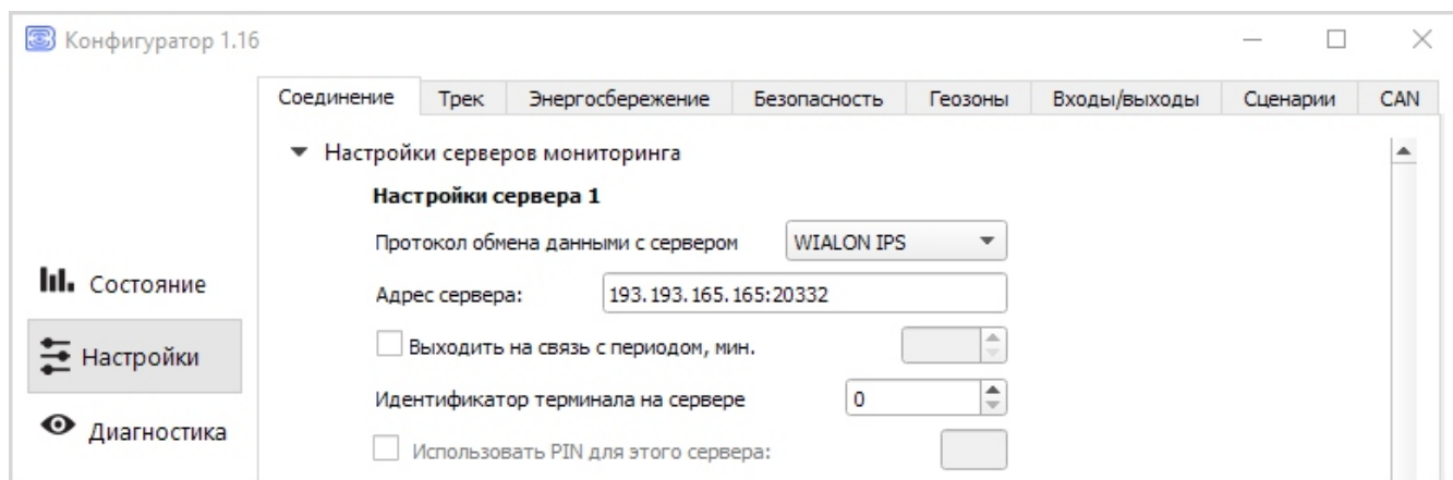
Рис. 5.2. Настройки серверов мониторинга.
