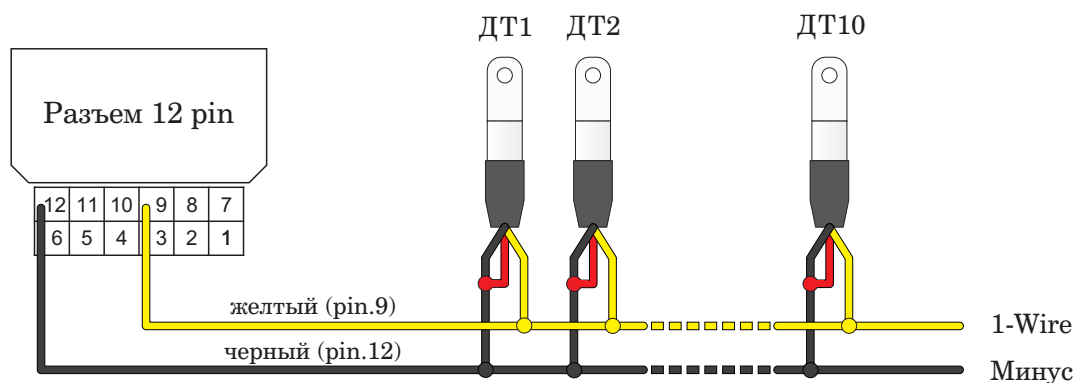
Рис. 4.1. Схема подключения датчиков температуры к шине 1-Wire.
