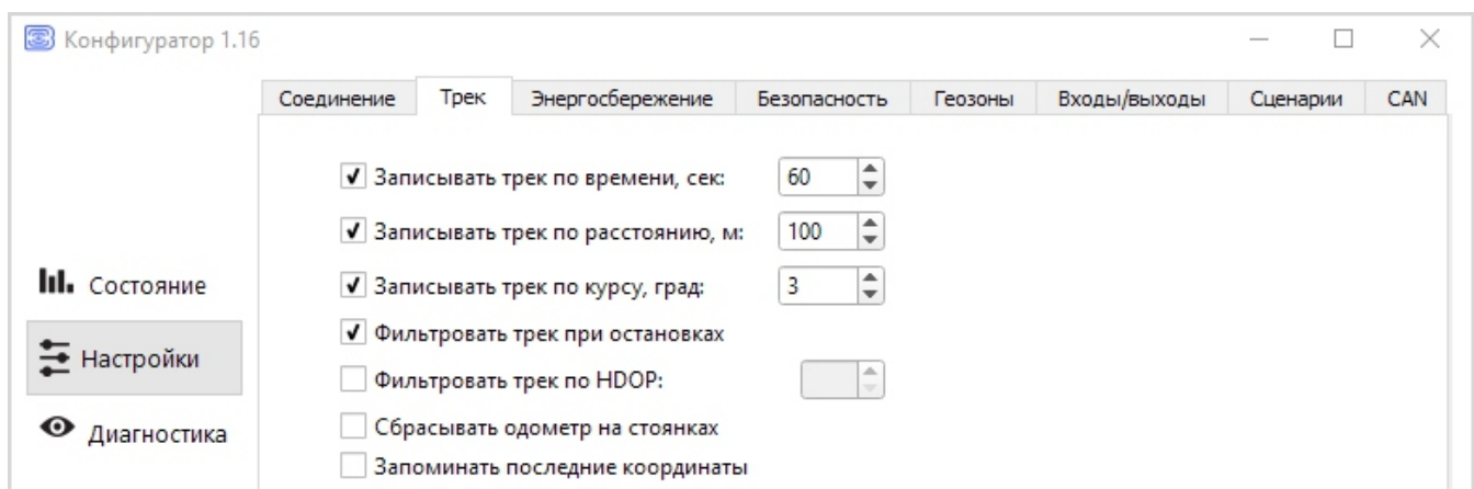
Рис. 5.5. Настройки вкладки «Треки».
