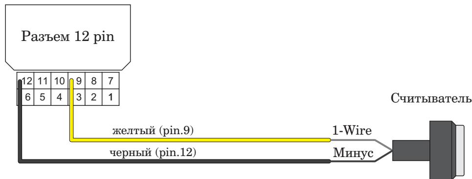
Рис. 4.3. Схема подключения считывателя авторизованных ключей к шине 1-Wire.
