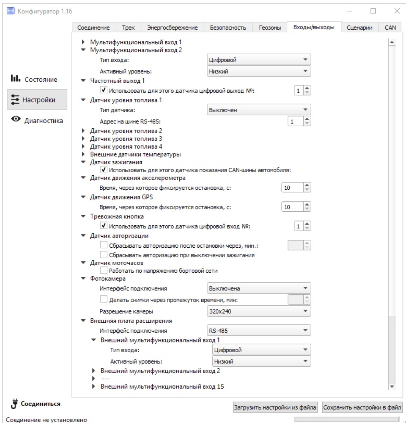
Рис. 5.9. Настройки вкладки «Входы/выходы».
