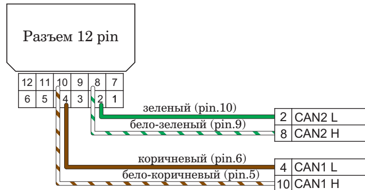
Рис. 4.5. Схема подключения к CAN-шине.
