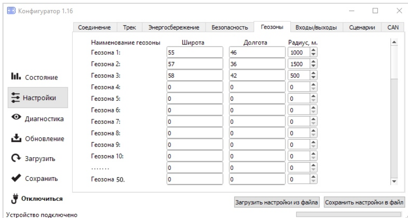
Рис.5.8. Настройки вкладки «Геозоны».
