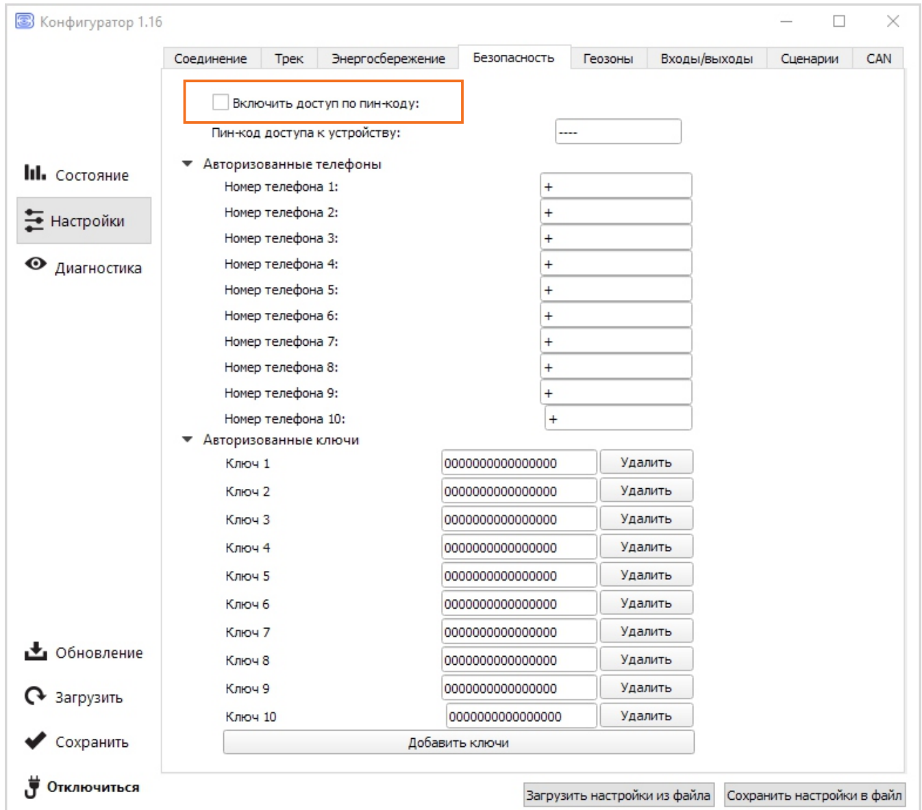
Рис. 5.7. Настройки вкладки «Безопасность».
