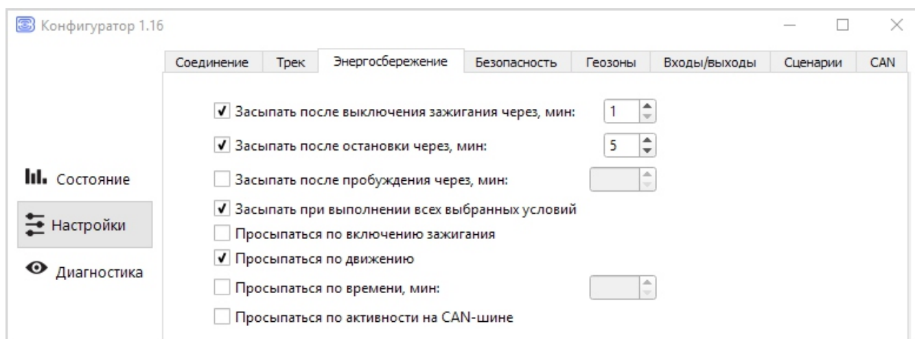
Рис. 5.6. Настройки вкладки «Энергосбережение».
