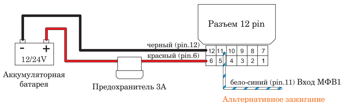
Рис. 3.3. Схема подключения питания.
