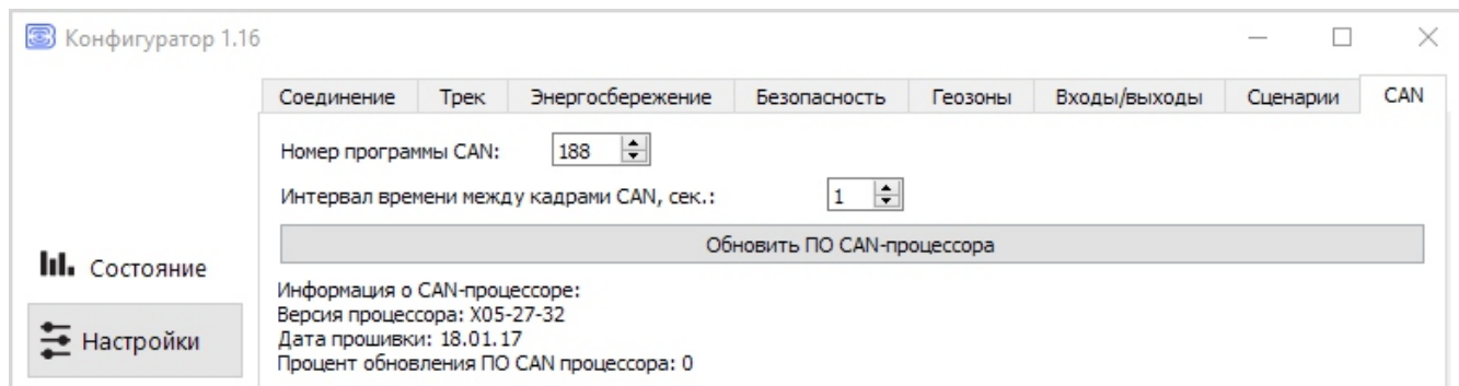
Рис. 5.11. Настройки для CAN-контроллера
