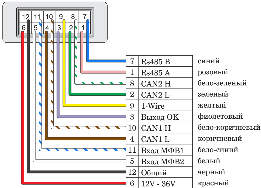
Рис. 3.2. Расположение контактов в разъеме.
