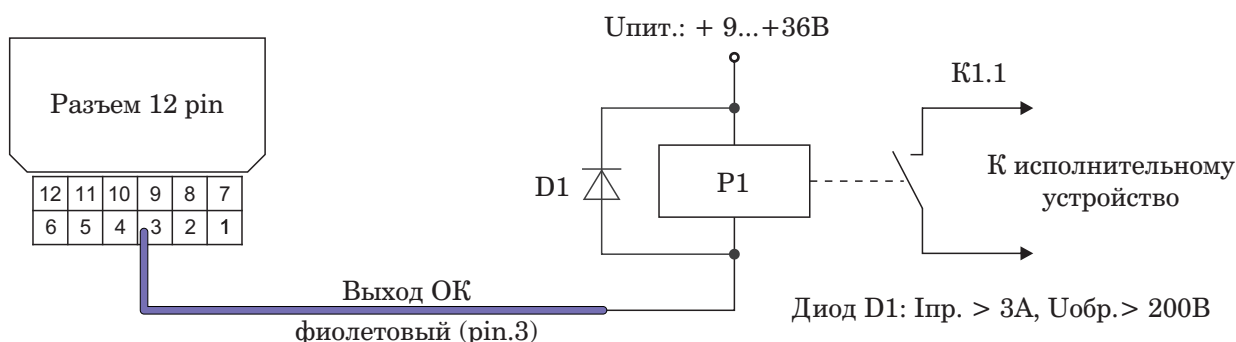
Рис. 4.7. Схема подключения реле на цифровой Выход ОК.
